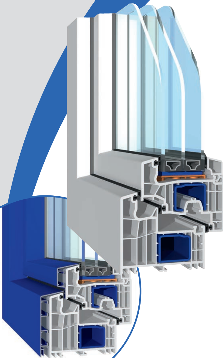
Alu-Vorsatzschale
